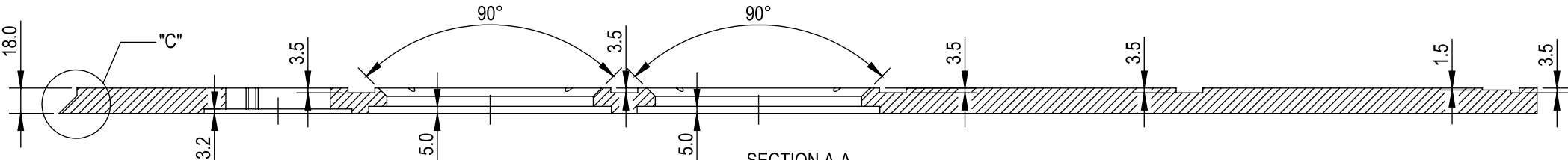
SECTION A-A SCALE 1 : 4
