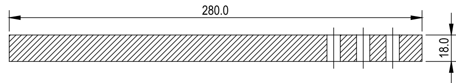
SECTION A-A SCALE 2 : 5
