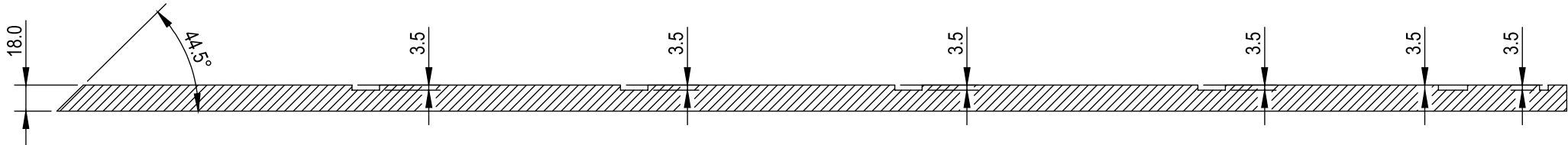
SECTION A-A SCALE 1 : 4
